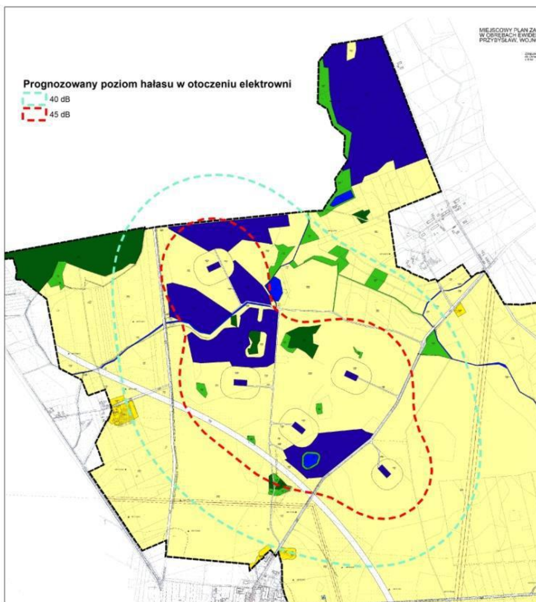
Ryc. 1. Zasięg izolacji w otoczeniu planowanej farmy wiatrowej na tle rysunku MPZP.
